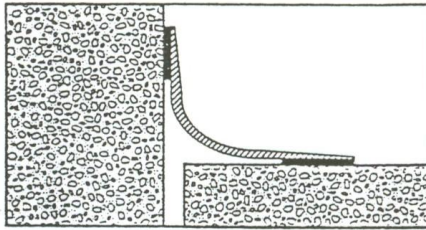
Zemin – duvar birleşim detayı
